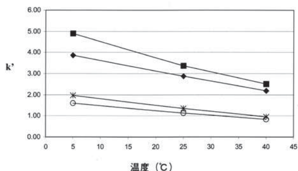
【図-2: 分離に対するカラム温度の影響】
