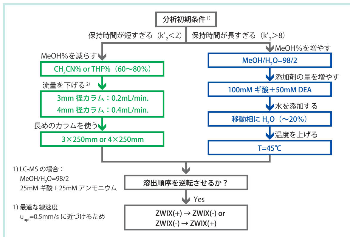
図1 分析条件決定フローチャート
